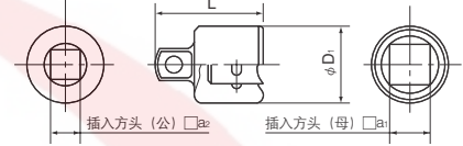
转接头
